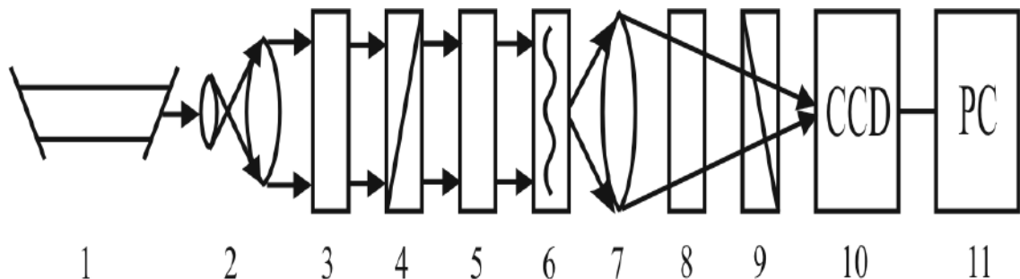
Рис. 1.1 Схема лазерного мікрополяриметра (CCD – charge-coupled device).
