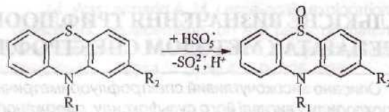
Рис. 1. Схема окиснення трифлюоперазину дигідрохлориду калію гідрогенпероксомоносульфатом.
