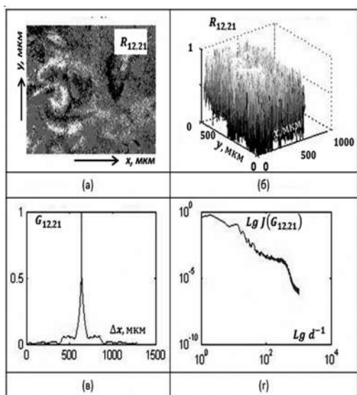
Рис. 7. Координатна (а), імовірнісна (б), кореляційна (в) та самоподібна (г) структура дійсної складової елемента матриці Джонса R_{12,21} полікристалічної мережі шару метіоніну.
