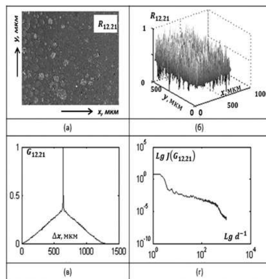
Рис. 8. Координатна (а), імовірнісна (б), кореляційна (в) та самоподібна (г) структура дійсної складової елемента матриці Джонса R_{12,21} полікристалічної мережі шару проліну.
