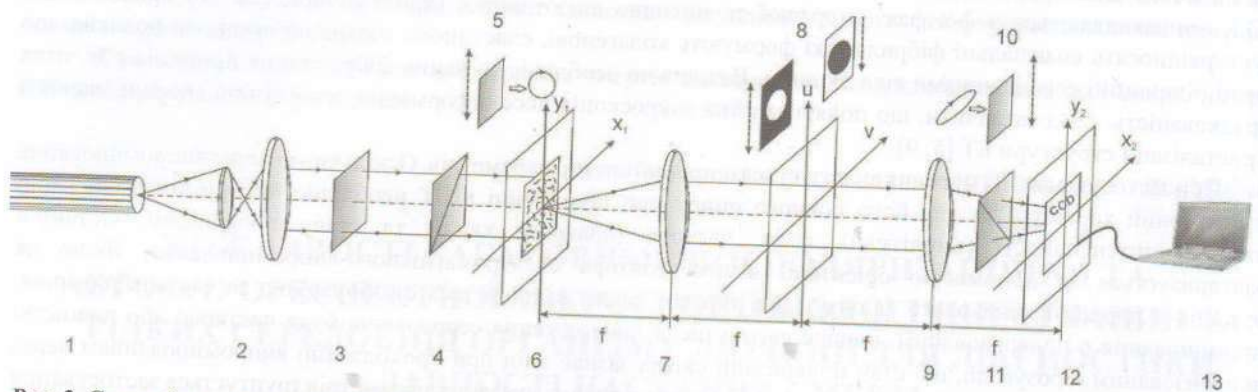
Рис. 2. Схема Стокс-поляриметра з використанням просторово-частотної фільтрації: 1 – He-Ne лазер; 2 – коліматор; 3 – стаціонарна чвертьхвильова платівка; 5, 10 – механічно рухомі чвертьхвильові платівки; 4, 11 – поляризатор та аналізатор; 6 – об'єкт дослідження; 7, 9 – поляризаційні мікрооб'єктиви; 8 – низькочастотний та високочастотний фільтри-діафрагми, 12 – CCD камера; 13 – персональний комп'ютер
