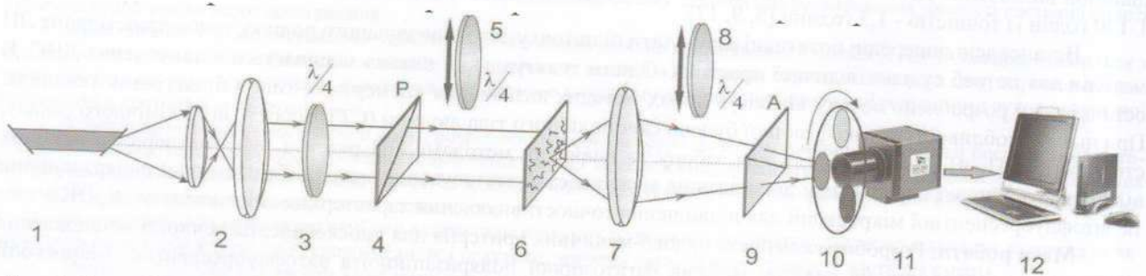
Рис. 3. Схема Стокс-поляриметра для дослідження автофлуоресценції біологічних шарів: 1 – He-Ne лазер; 2 – коліматор; 3 – стаціонарна чвертьхвильова платівка; 5, 8 – механічно рухомі чвертьхвильові платівки; 4, 9 – поляризатор та аналізатор; 6 – об'єкт дослідження; 7 – поляризаційний мікрооб'єктив; 11 – CCD камера; 12 – персональний комп'ютер.
