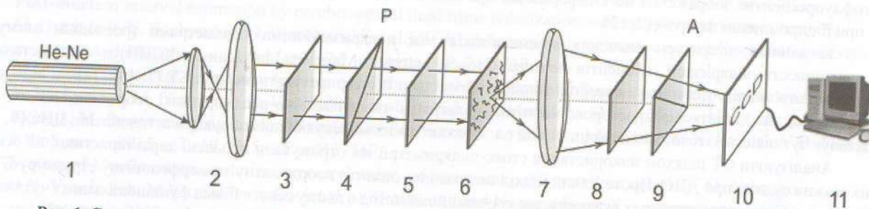
Рис. 1. Схема стандартного Стокс-поляриметра: 1 – He-Ne лазер; 2 – коліматор; 3,5,8 – стаціонарні чвертьхвильові платівки; 4, 9 – поляризатор та аналізатор; 6 – об'єкт дослідження; 7 – поляризаційні мікрооб'єкти; 10 – CCD камера; 11 – персональний комп'ютер.
