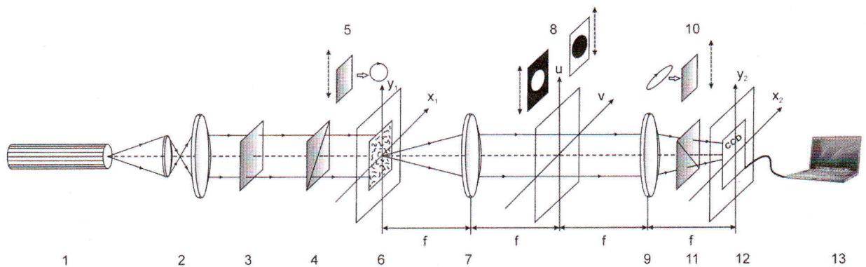
Рис. 1. Оптична схема стокс-поляриметра з використанням просторово-частотної фільтрації, де
